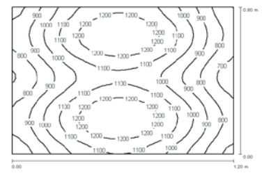
SLE / SLZE 2x39W T5 E_{max} = 1306 \text{ lx}
